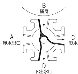
2. 逆洗狀態
