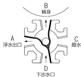
1. 濾水狀態
